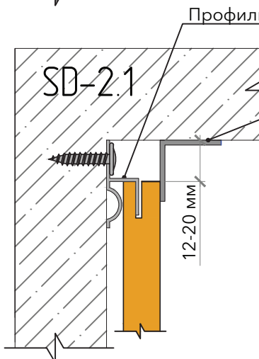
Декоративный алюминиевый шпонируемый уголок 25x25
